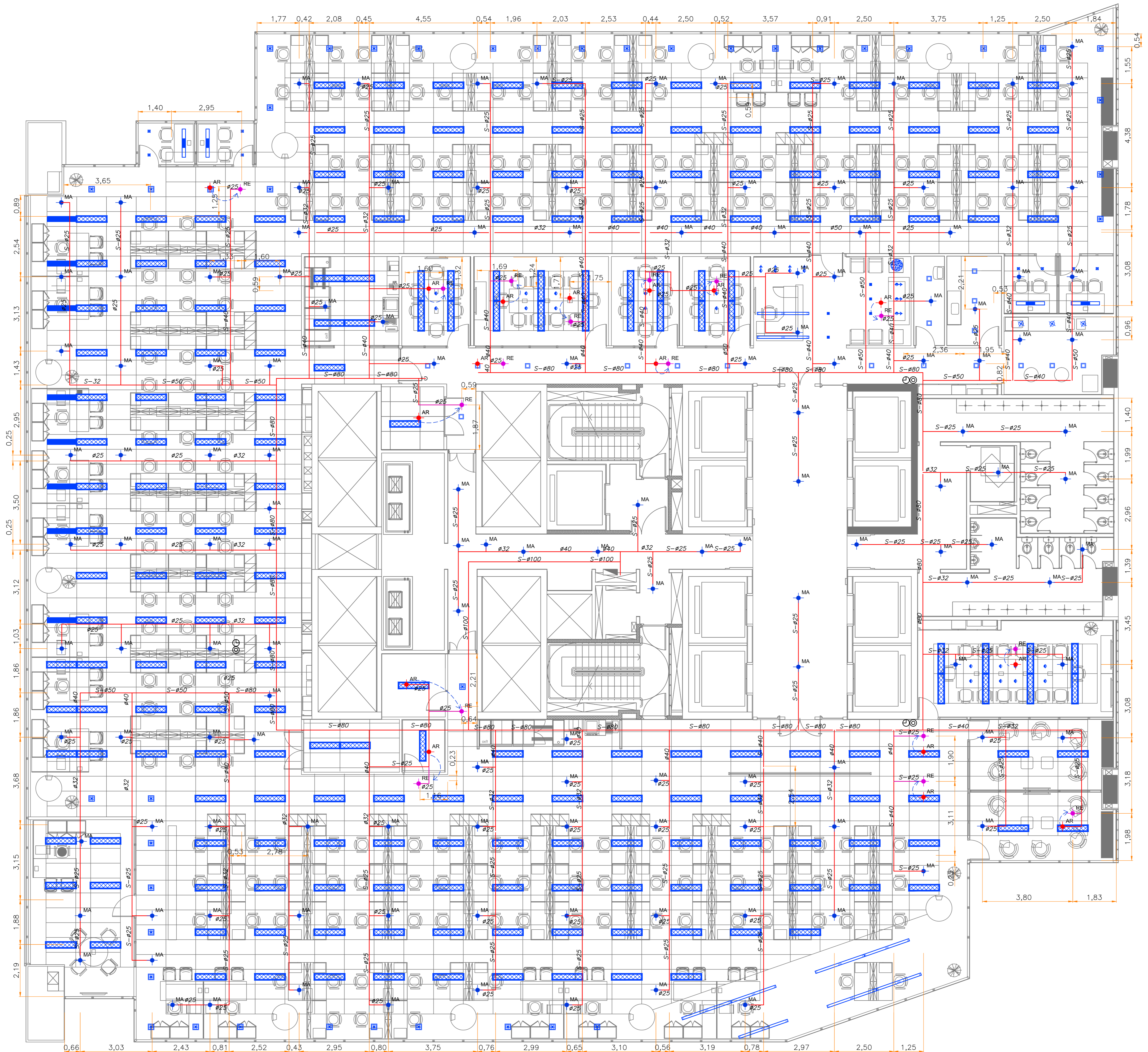
16º PAVIMENTO PLANTA ESCALA 1:75
